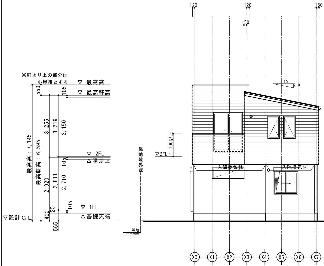
南側立面図 S:1/100
