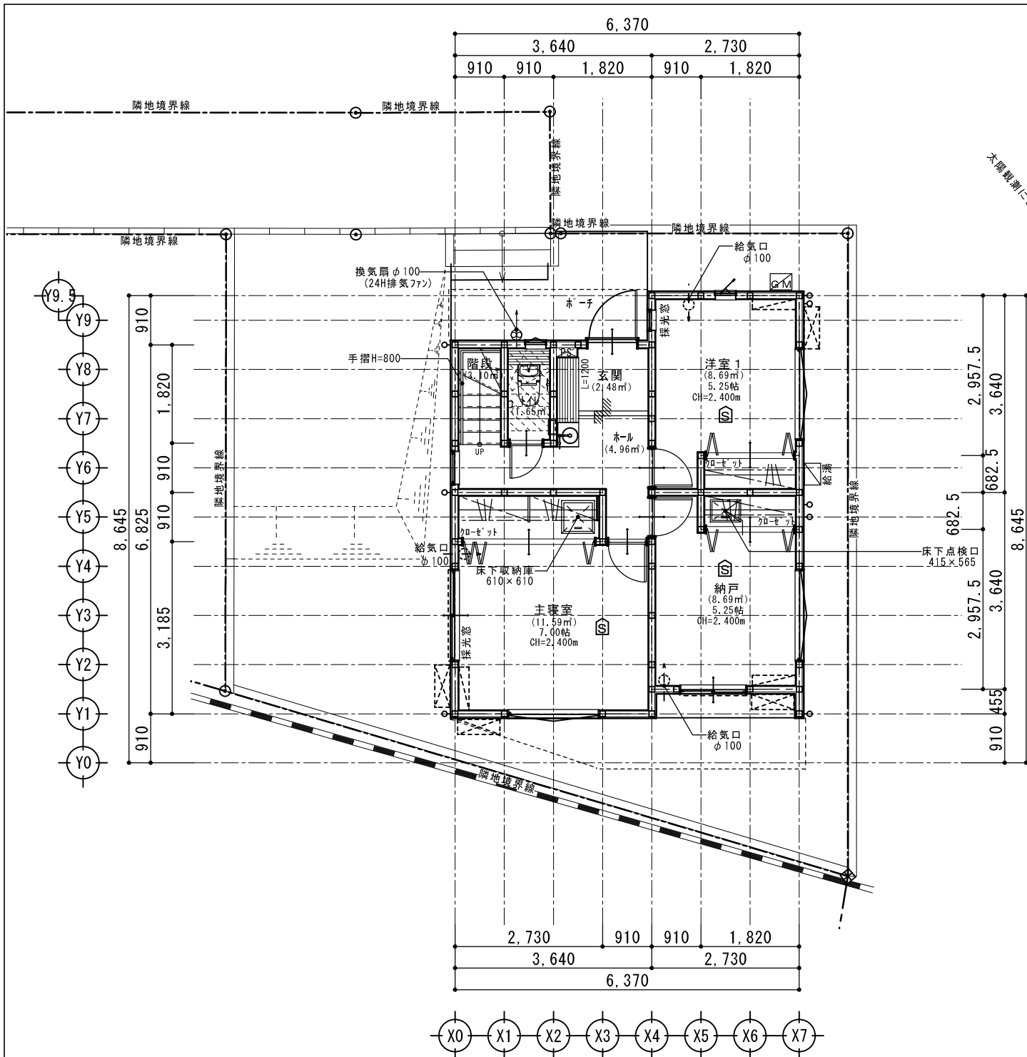
1階平面図 S:1/100
