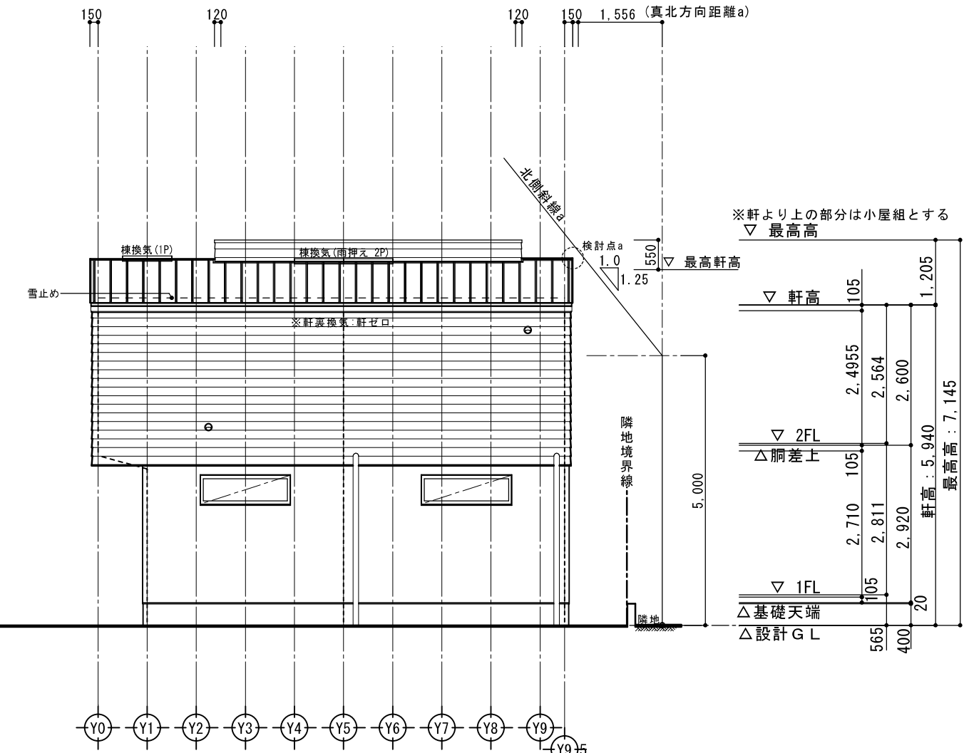
東側立面図 S:1/100
