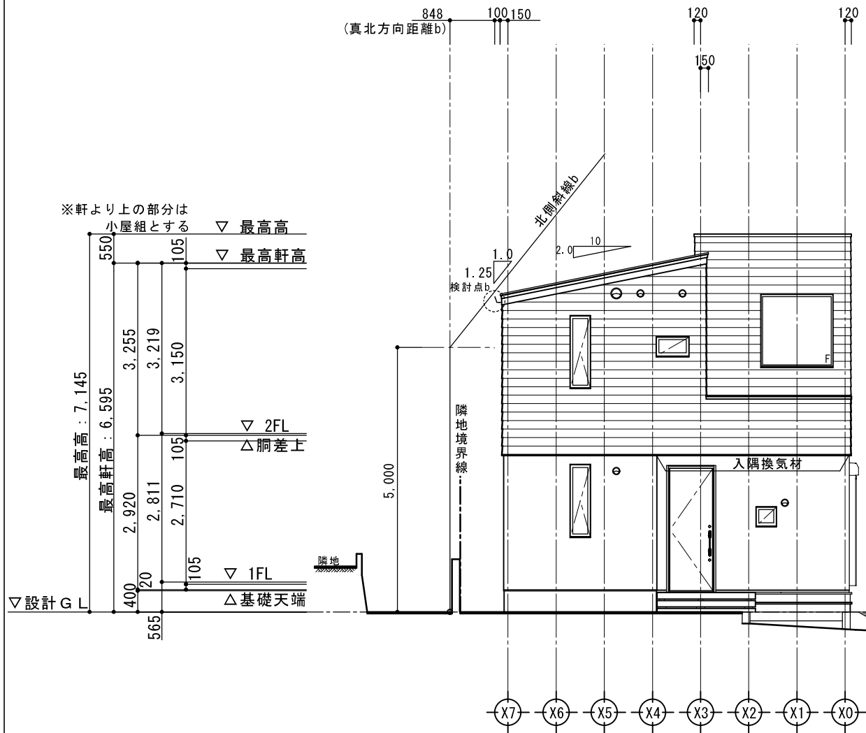
北側立面図 S:1/100
